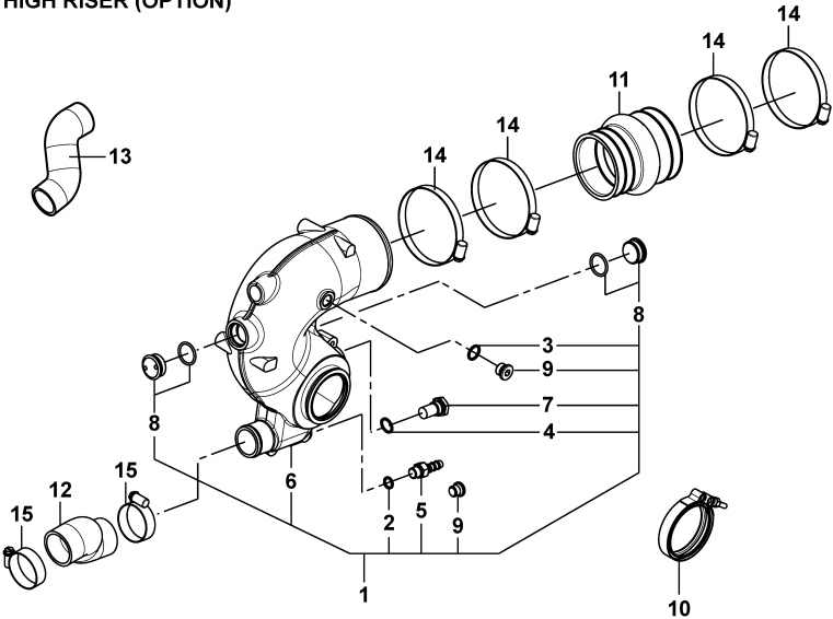
ハイライザー (オプション) HIGH RISER (OPTION)
